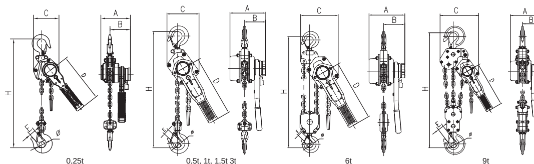
Fig. 1 Maattekening
