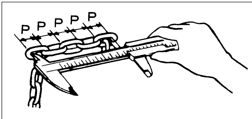
Рис. 5 Проверка цепи
