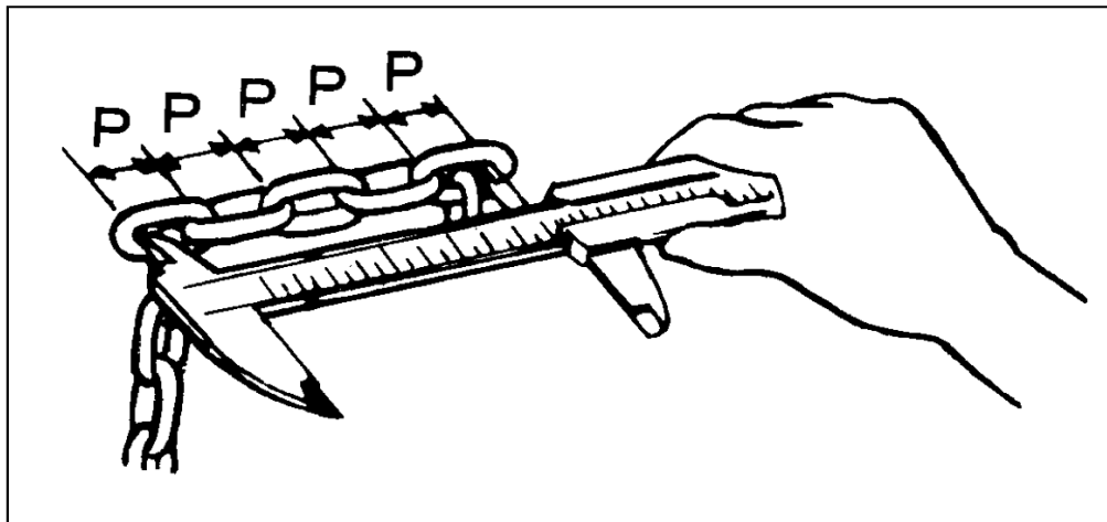
Kuva 5 Kuormaketjun kontrollimittaus
