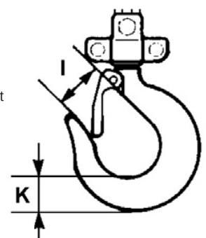
Abb. 4 Lastenhaken
